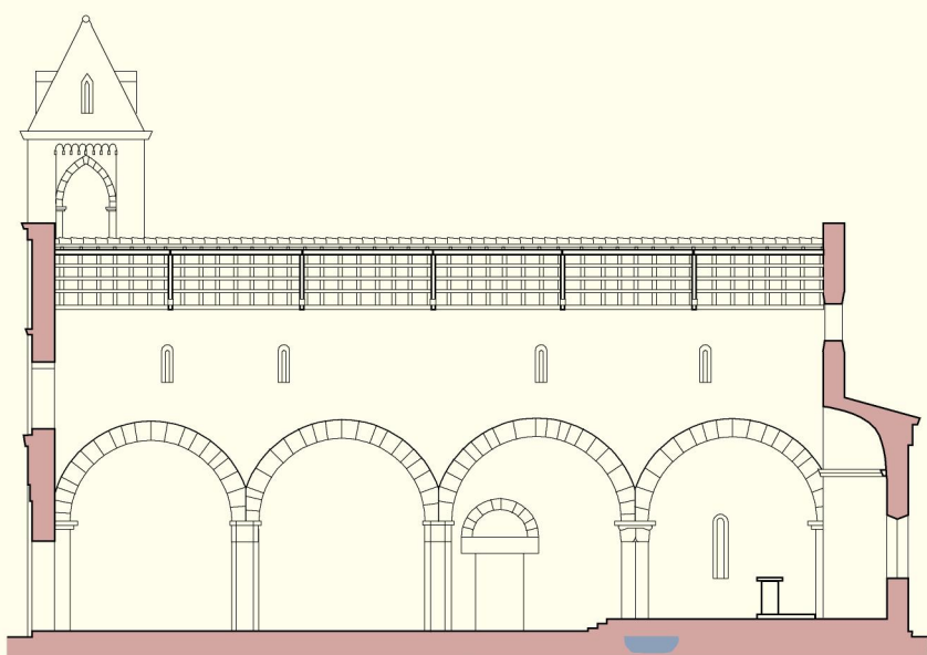
Sezione longitudinale
