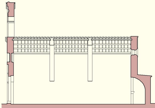
Sezione longitudinale
