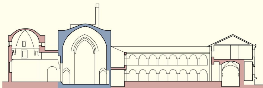
Sezione trasversale
