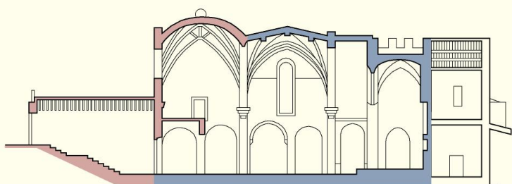
Sezione longitudinale
