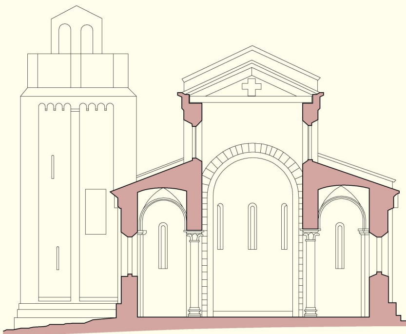
Sezione trasversale
