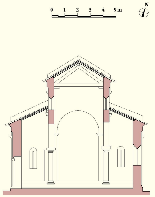
Sezione trasversale
