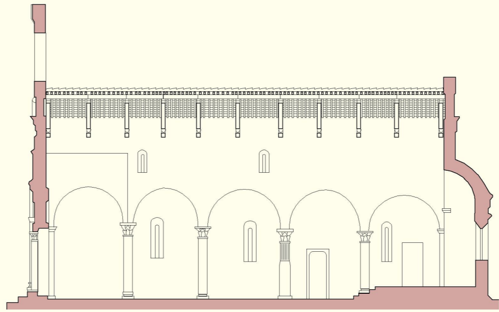
Sezione longitudinale
