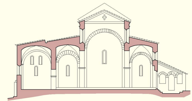
Sezione trasversale del transetto
