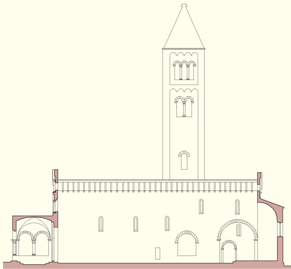
Sezione longitudinale
