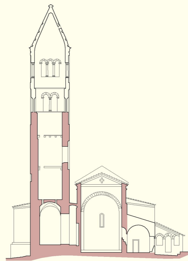
Sezione trasversale dell'aula e del campanile
