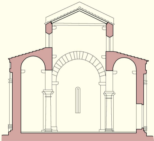
Sezione trasversale
