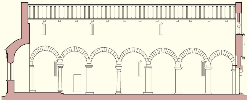
Sezione longitudinale
